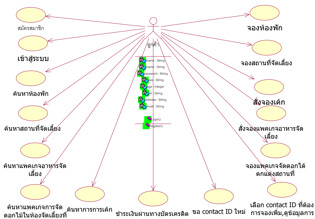
รูปที่ 8-3 Use Case Diagram ระบบโรงแรม (ส่วนที่ 1)
