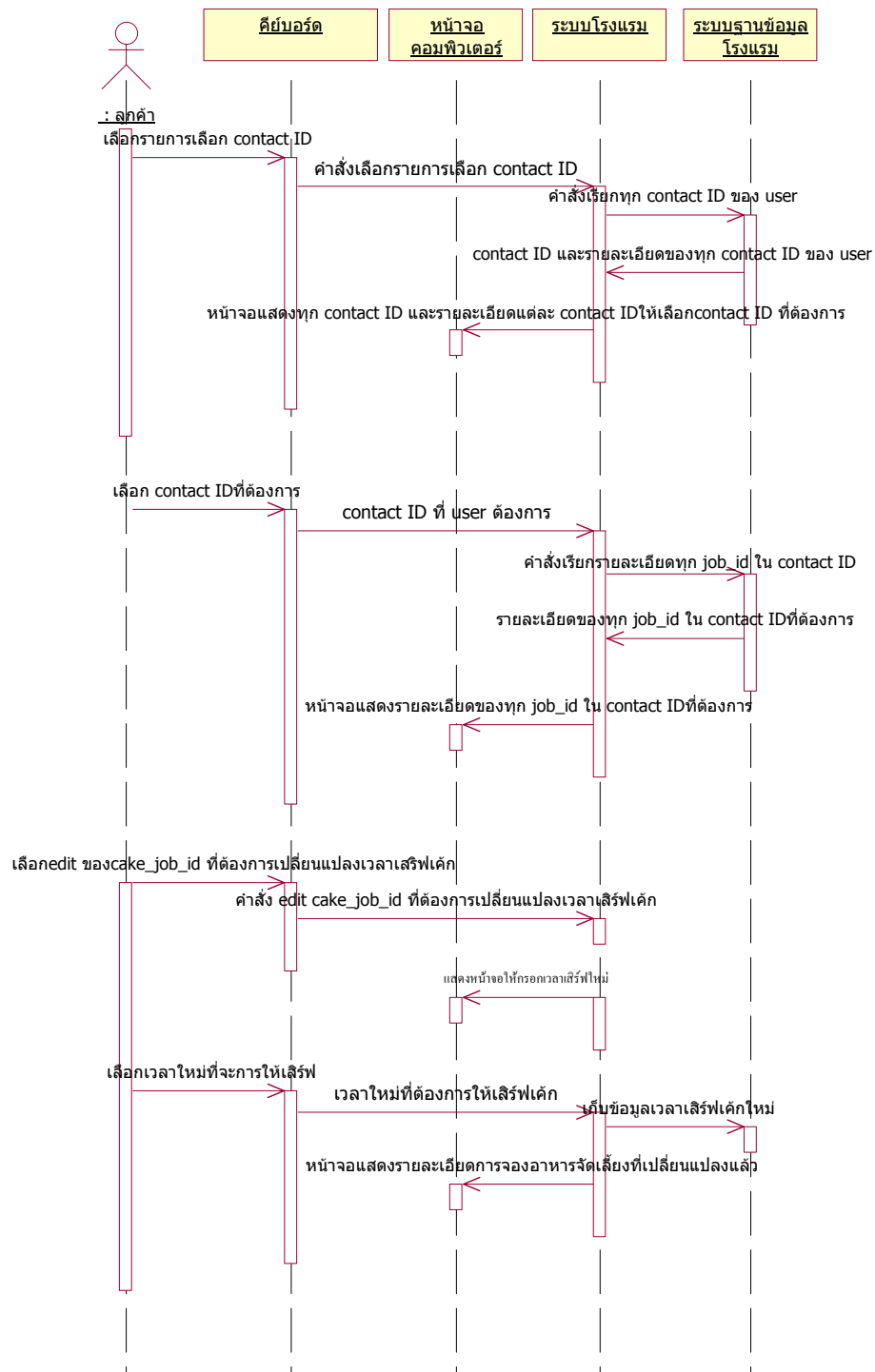
รูปที่ 8-27 Sequence Diagram การเปลี่ยนแปลงเวลาเสิร์ฟเค้ก ของระบบโรงแรม
