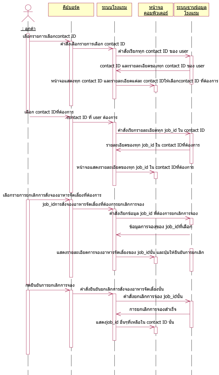
รูปที่ 8-32 Sequence Diagram การยกเลิกการจองอาหารจัดเลี้ยง ของระบบโรงแรม
