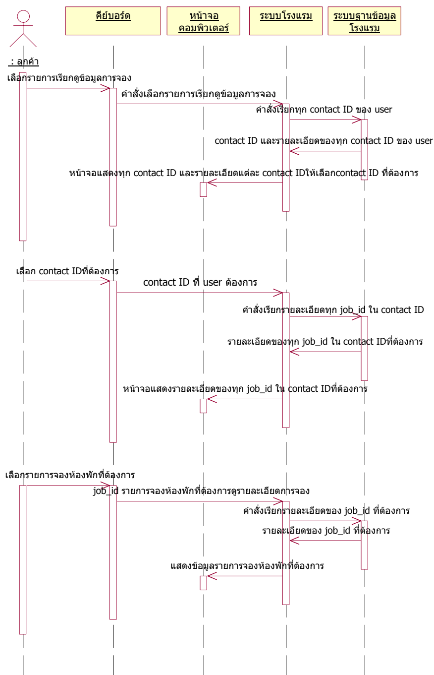
รูปที่ 8-20 Sequence Diagram การเรียกดูข้อมูลการจองห้องพักที่ต้องการ ของระบบโรงแรม
