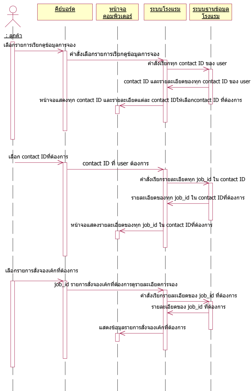
รูปที่ 8-24 Sequence Diagram การเรียกดูข้อมูลการสั่งเค้ก
