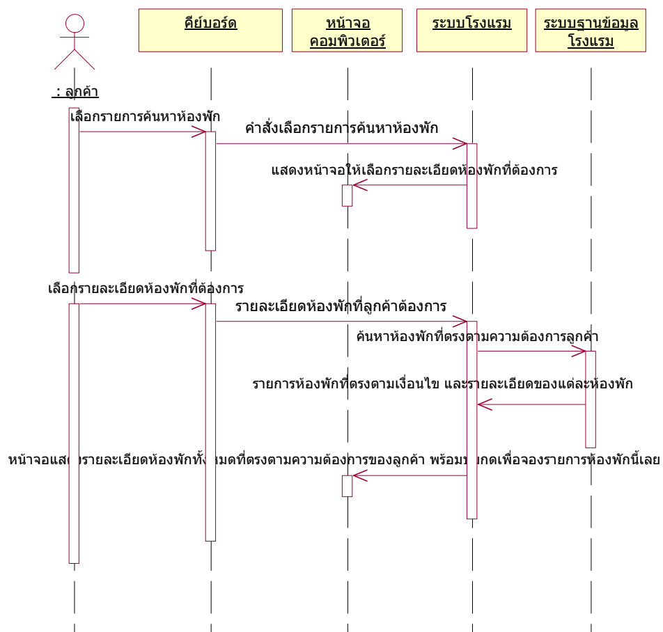
รูปที่ 8-7 Sequence Diagram การค้นหาห้องพัก ของระบบโรงแรม
