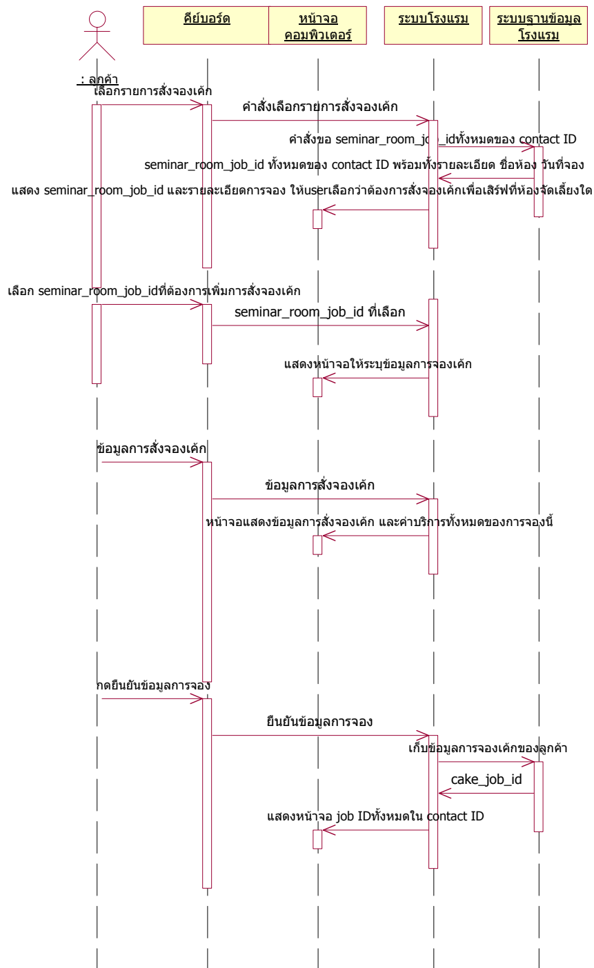
รูปที่ 8-15 Sequence Diagram การสั่งจองเค้กของระบบโรงแรม
