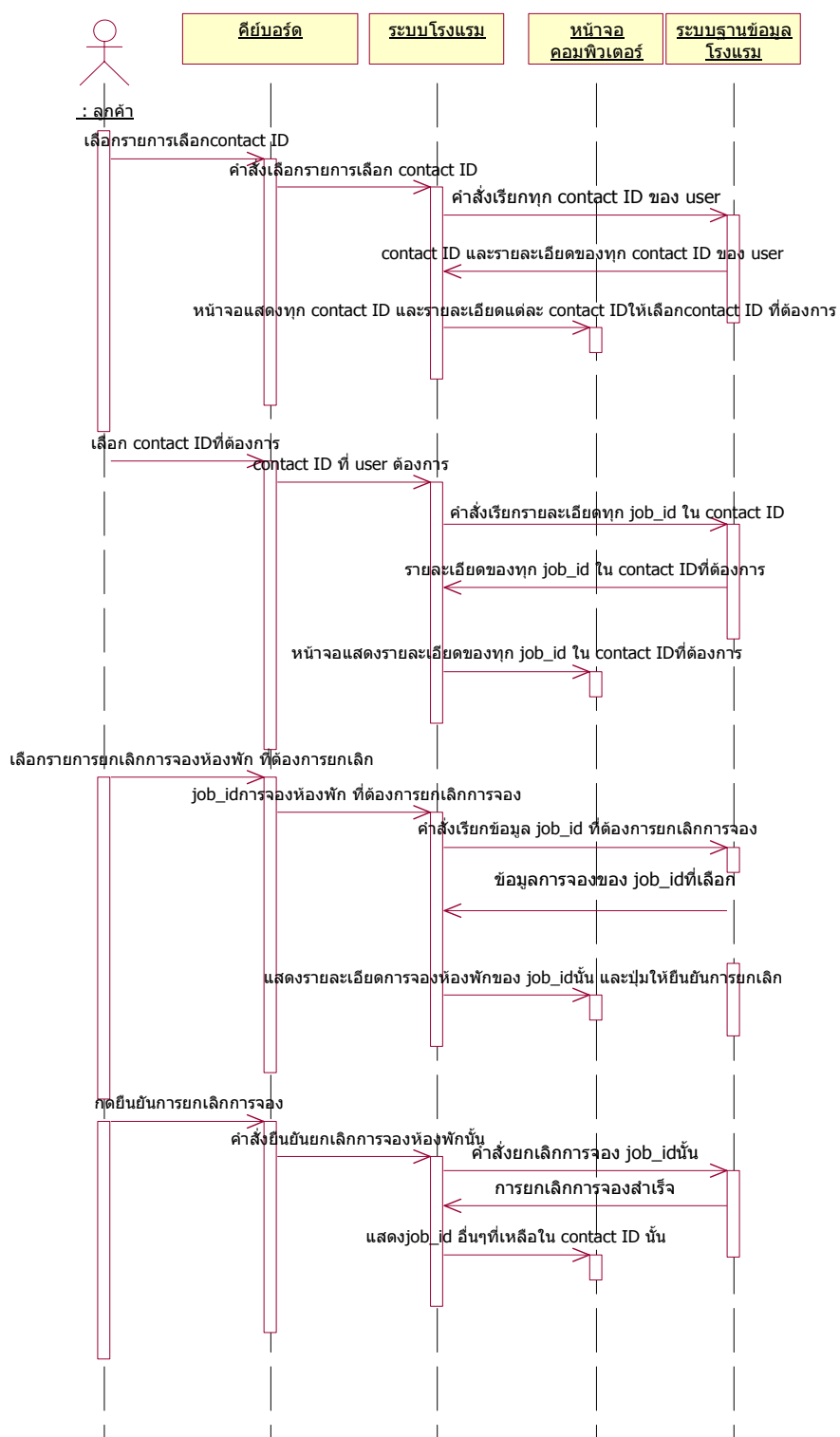
รูปที่ 8-29 Sequence Diagram การยกเลิกการจองห้องพักของระบบโรงแรม
