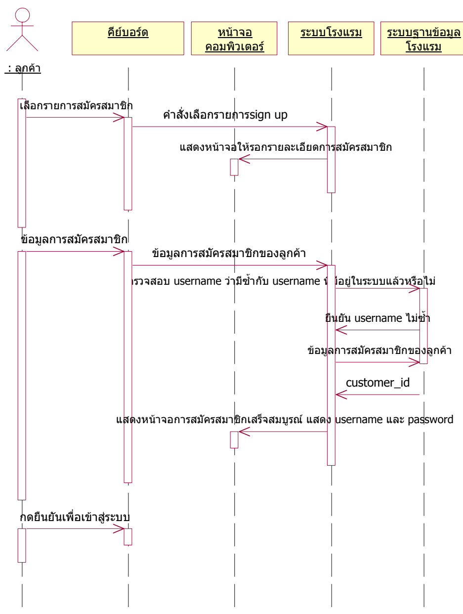
รูปที่ 8-5 Sequence Diagram การสมัครสมาชิก ของระบบโรงแรม
