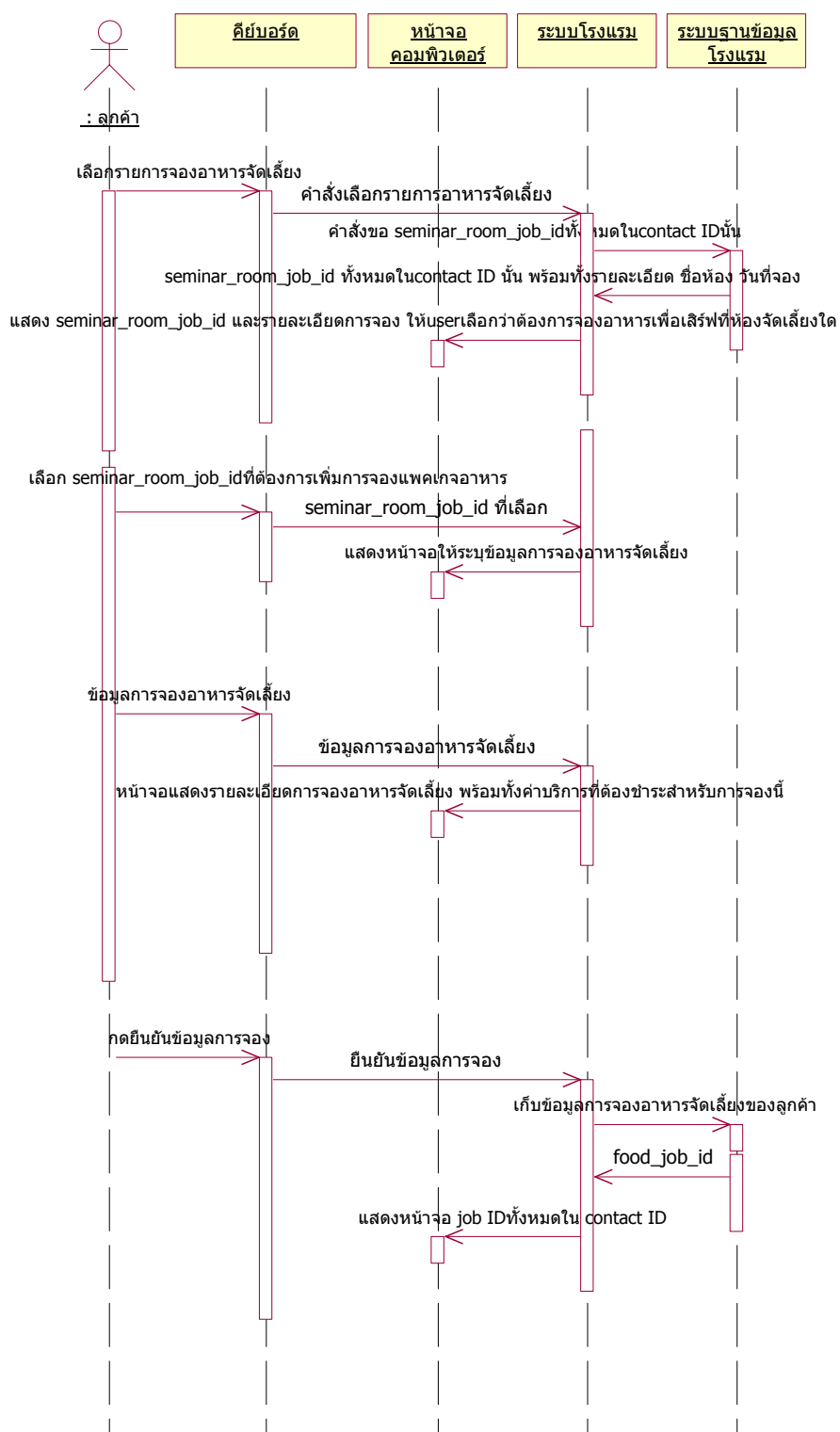
รูปที่ 8-14 Sequence Diagram การจองแพคเกจอาหารจัดเลี้ยง ของระบบโรงแรม
