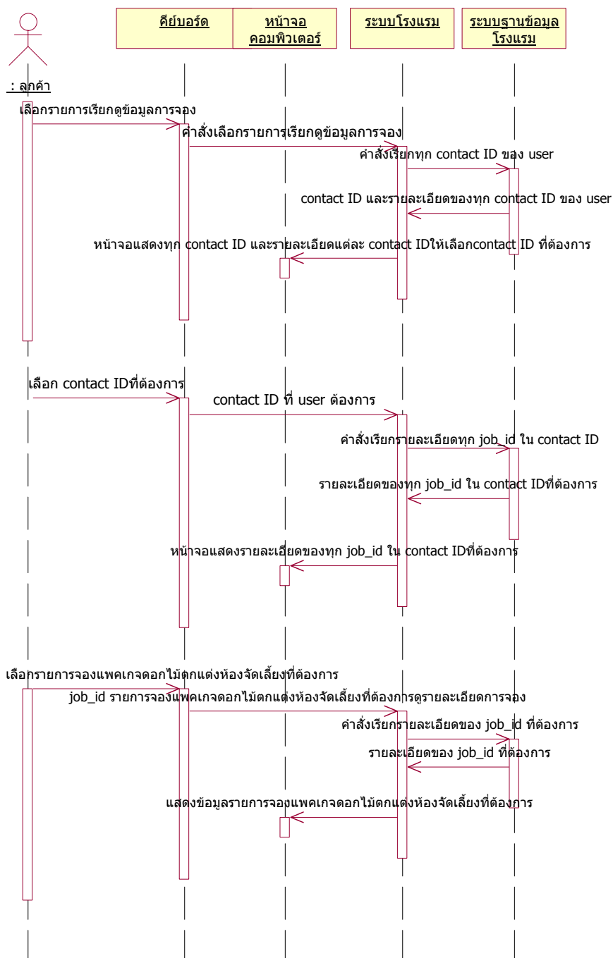
รูปที่ 8-22 Sequence Diagram การเรียกดูการจองแพคเกจดอกไม้ตกแต่งห้องจัดเลี้ยง
